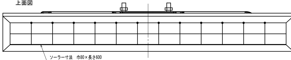
上面図
