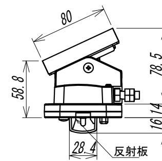
側面図（出荷時）
