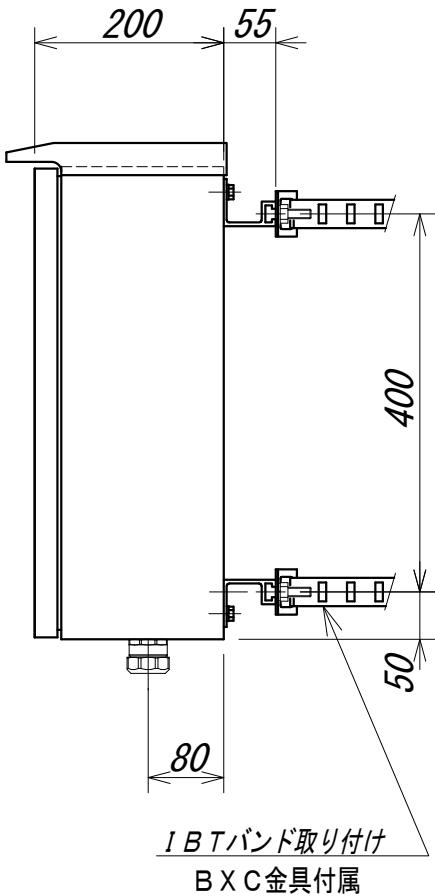
側面図
