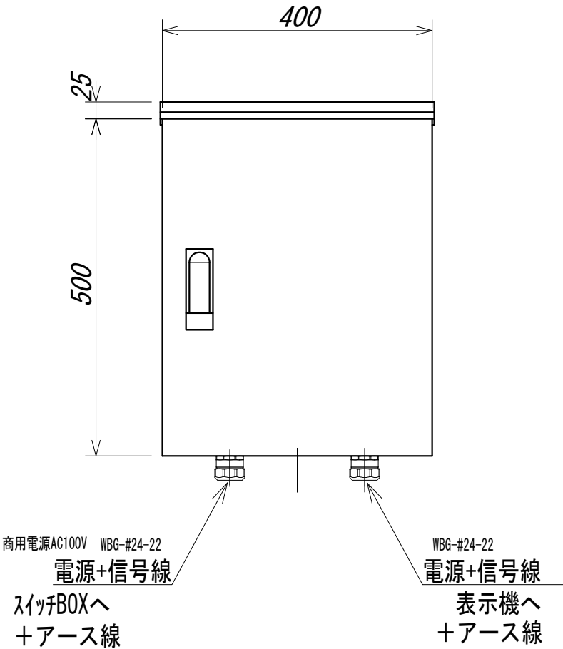
正面図
