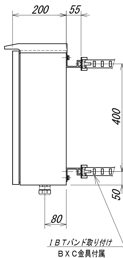
側面図
